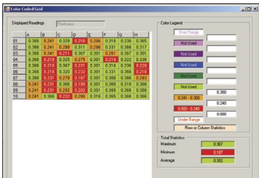
Выводимая на экран компьютера таблица значений с цветовыми кодами наглядно отображает участки с толщиной, не соответствующей допускам.
