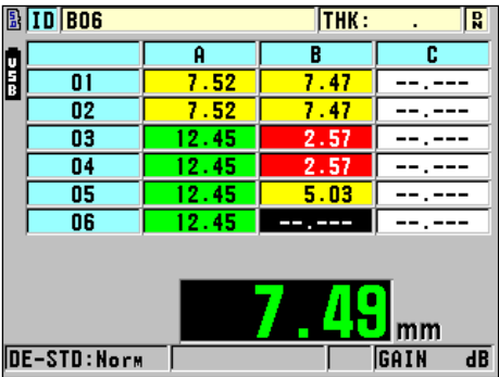
Отображаемая на экране прибора таблица значений с тремя задаваемыми цветовыми кодами
